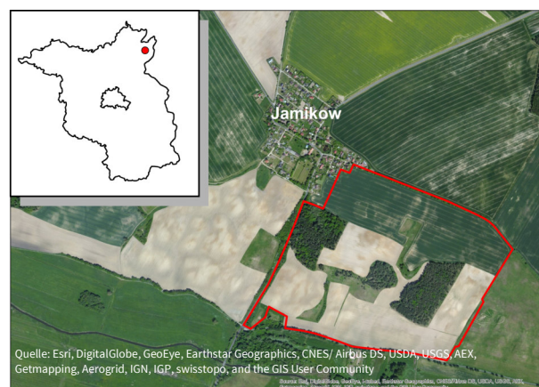
Naturschutzgebiet Trockenrasen Jamikow mit Lage in Brandenburg
