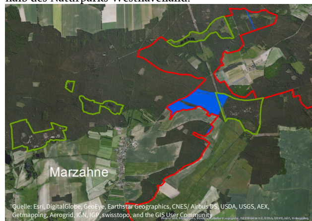
Marzahner Fenn und Dünenheide (blau) als Teil eines Vogelschutzgebietes (rot) und FFH-Gebietes (grün)
